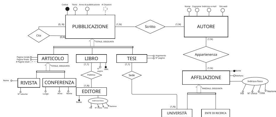
Figura 3: Schema Entità-Relazione
